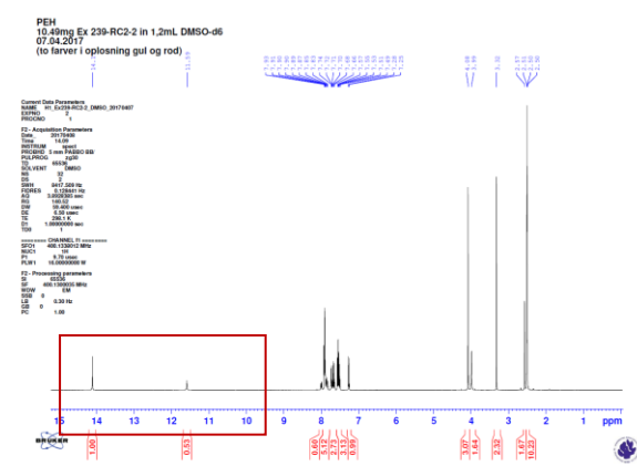
Фиг. 11. ^1\text{H} NMR спектър на 3.2 в \text{DMSO-}d_6 .
