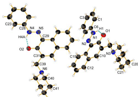
Фиг.6. Кристална структура на 2.3.
