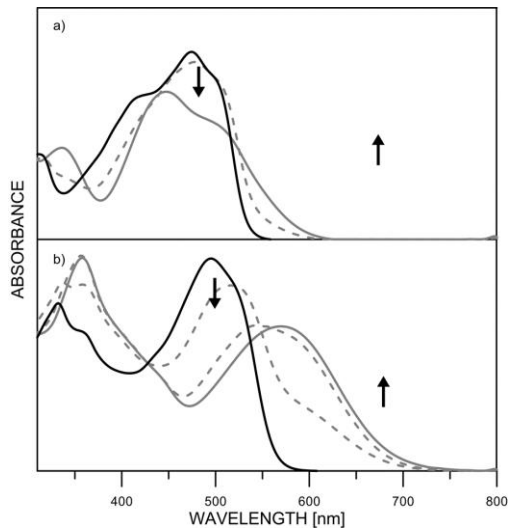
Фиг. 4. Абсорбционен спектър на а) 2.1 и б) 2.2 в ACN при добавяне на база: (— без добавяне на база; — крайен спектър при добавяне на база).
