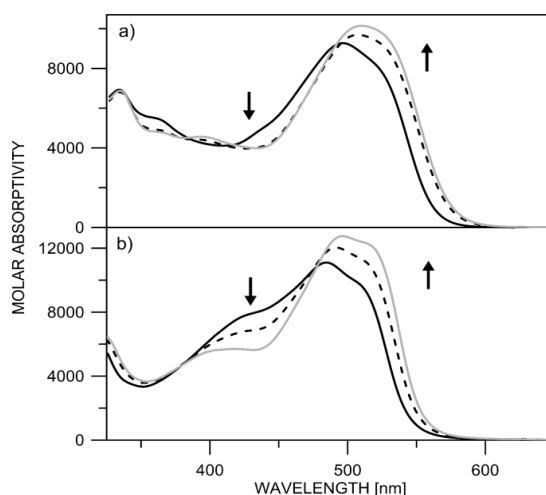
Фиг. 2. Абсорбционни спектри на а) 2.2 в ACN и б) 2.3 в DMSO, при добавяне на вода: (— без добавена вода; — краен спектър при добавена вода).
