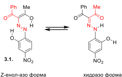
Схема 3. Тавтомерно равновесие при 3.1 .
