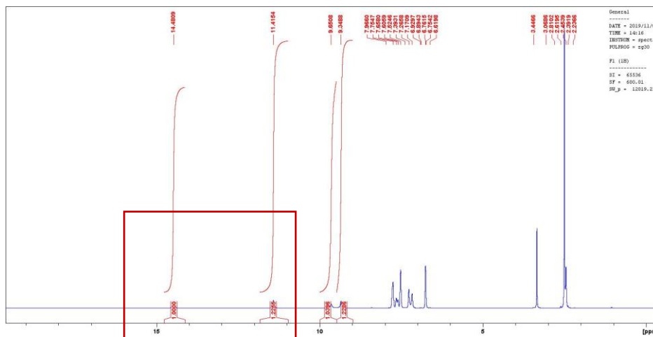
Фиг. 32. ^1\text{H} NMR спектър на 3.4 в \text{DMSO-d}_6 .
