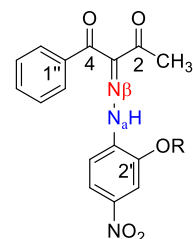
Схема 5. Номериране на въглеродните атоми при 3.1 (R=H) и 3.2 (R=CH 3 ).
