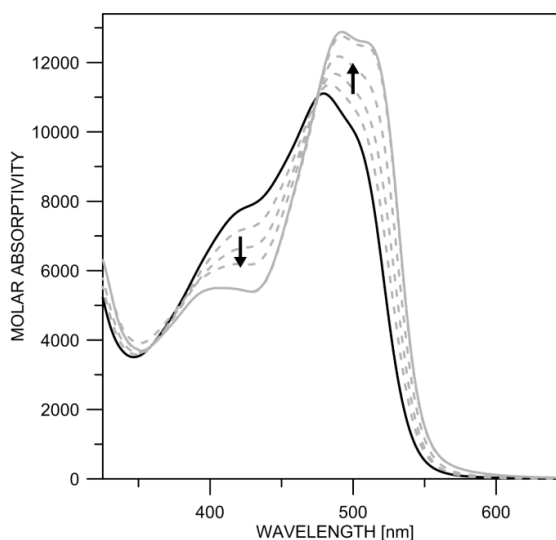
Фиг.7. Абсорбционни спектри на 2.3 в ACN при добавяне на киселина: (—без добавяне на киселина; ---краен спектър след добавяна киселина).
