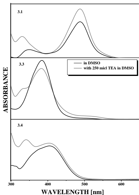
Фиг. 33. Промяна в абсорбционния спектър на 3.1 , 3.3 и 3.4 в DMSO при добавяне на триетиламин ( TEA ) ( 250 \mu\text{l TEA} съответства на 4 \times 10^3 екв).
