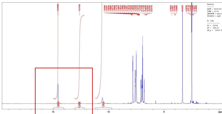
Фиг. 31. ^1\text{H} NMR спектър на 3.3 в \text{DMSO-d}_6 .
