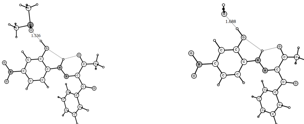
Фиг. 20. Комплекси на 3.1E' с DMSO (ляво) и с вода (дясно). Дължината на междумолекулната водородна връзка е дадена в Å.
