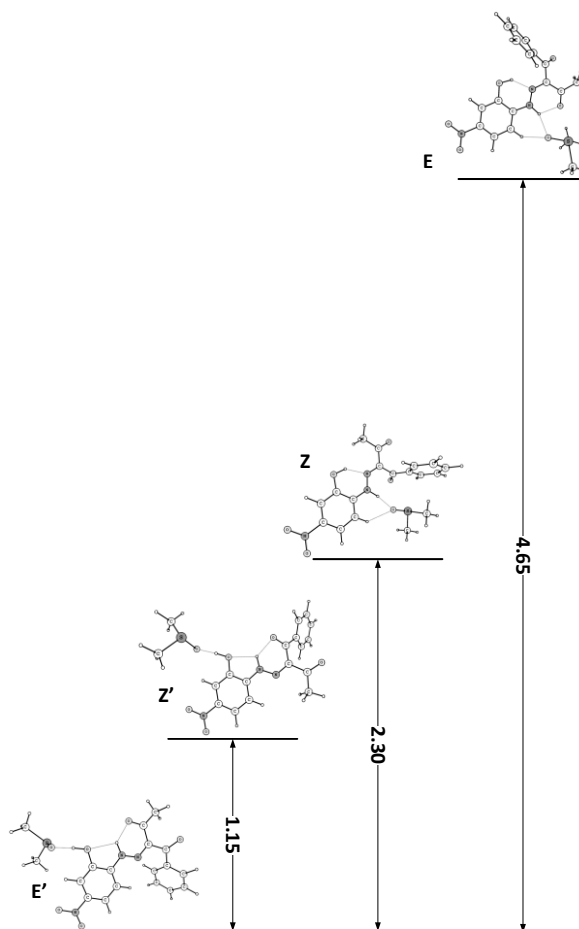
Фиг. 13. Относителни енергии (в kcal/mol) на най-стабилните конформационни изомери на 3.1I в DMSO, отчитайки специфичното взаимодействие с разтворителя.
