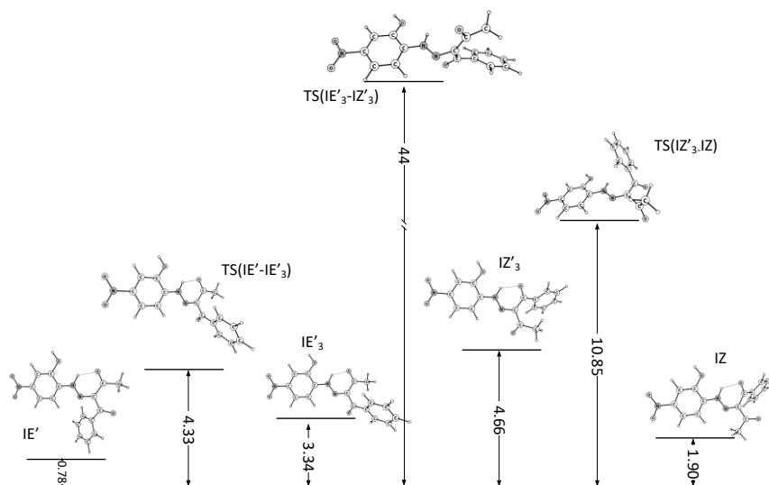
Фиг. 15. Енергетична диаграма на прехода от 3.IE' към 3.IZ' и обратно в DMSO (показаните стойности са представени в kcal/mol ).
