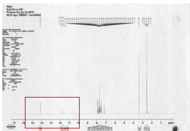
Фиг. 10. ^1\text{H} NMR спектър на 3.1 в \text{DMSO-}d_6 .
