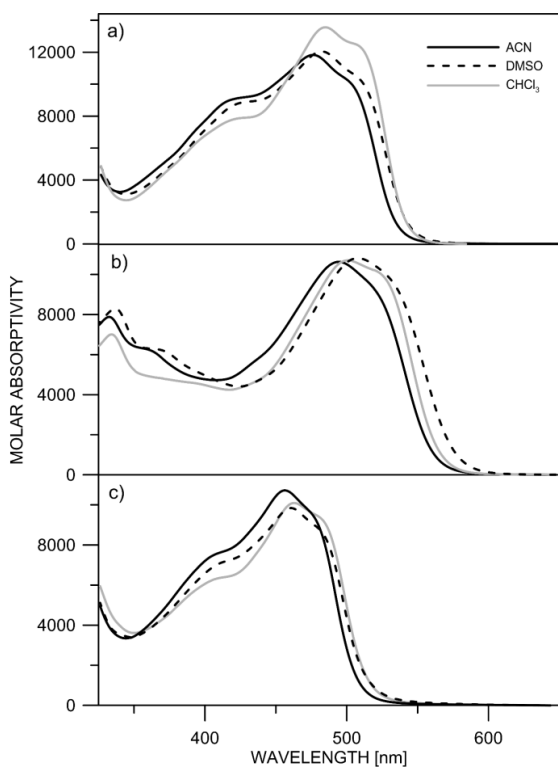
Фиг. 1. Абсорбционни спектри на а) 2.1 , б) 2.2 и с) 2.3 в различни разтворители.
